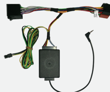
Faisceau CANBUS Valtra
