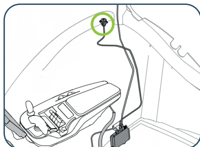
TERMINAL SMART TOUCH branchement sur prise 7 voies AMP sur la console
